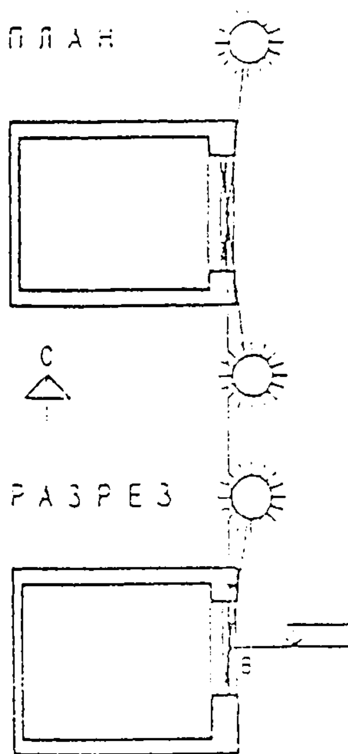
Рис. 1. Схема определения расчетной точки для окна.
